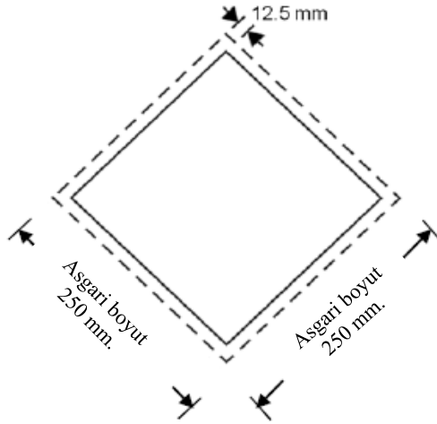
Şekil 5.3.1.7.1 Levha (Sınıf 7 Hariç)
