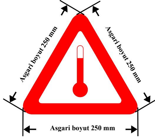
Şekil 5.3.3 Yüksek Sıcaklıkta Taşıma İşareti
